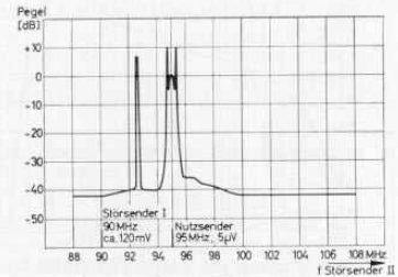
B) Großsignalverhalten FM (Mehrfachempfangsstellen) mit 2 Störsendern. Nutzsender: 5 \mu\text{V} an 300 \Omega , 95 \text{ MHz} , unmoduliert Störsender I: ca. 120 \text{ mV} an 300 \Omega , 90 \text{ MHz} , 1 \text{ kHz} NF \pm 40 \text{ kHz} Hub. Störsender II: 100 \text{ mV} an 300 \Omega , 88 - 108 \text{ MHz} , 1 \text{ kHz} NF \pm 40 \text{ kHz}
