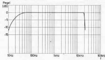
I) Frequenzgang TA-Magnet (über Schneidkennlinien-Nachbildung) mit steilem Abfall der Frequenzen unterhalb 40 Hz (Rumpffrequenzen), gemessen am Lautsprecherausgang
