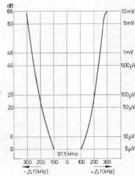
D) Dynamische Selektion, Mono Nutzsender: 5 \mu\text{V} an 300 \Omega , 97,5 \text{ MHz} unmoduliert. Störsender: 1 \text{ kHz} \pm 40 \text{ kHz} Hub. Messung: 30 \text{ dB} Störabstand bezogen auf Nutzsignal von Nutzsender bei 1 \text{ kHz} \pm 40 \text{ kHz} Hub, gemessen von 31,5 \text{ Hz} - 15 \text{ kHz} , effektiv.
